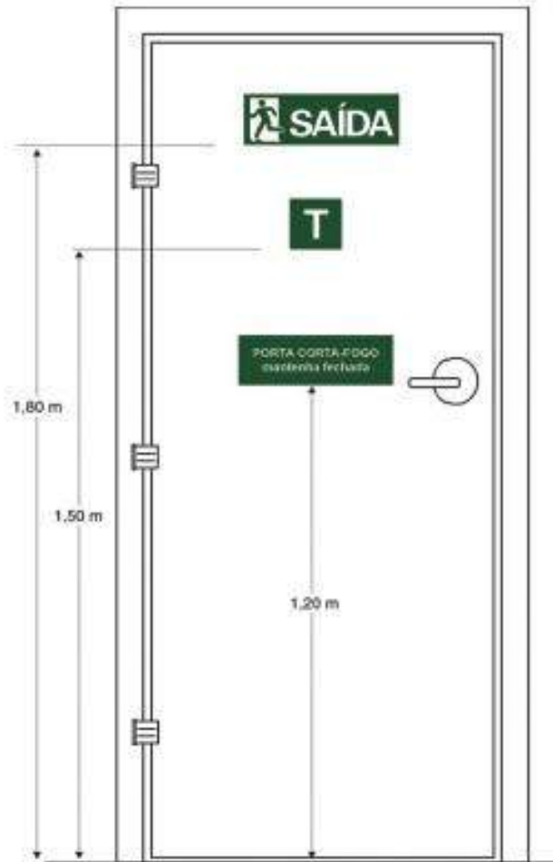
Figura 221. Sinalização de porta corta-fogo
