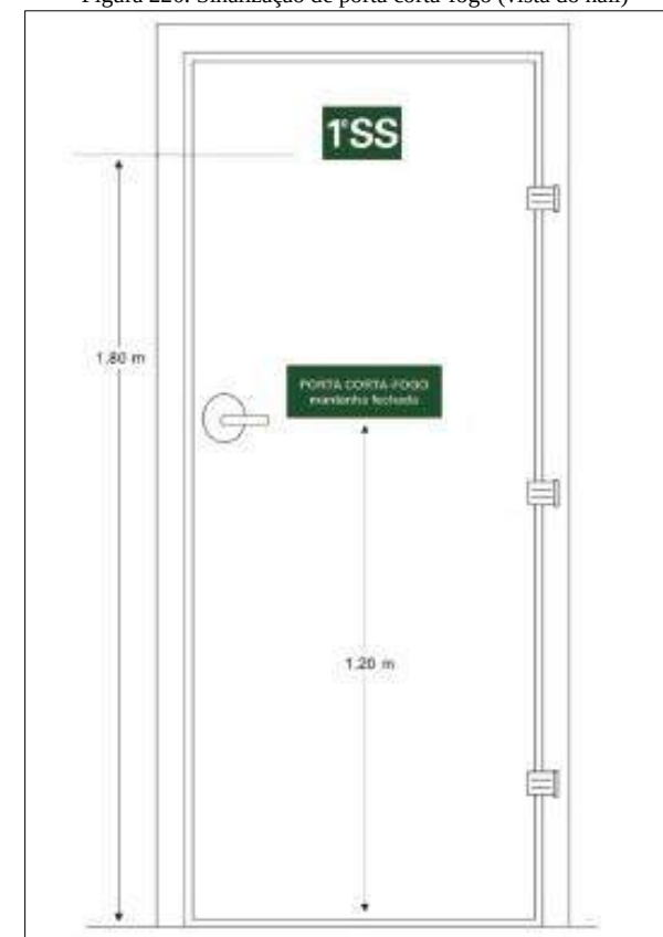
Figura 220. Sinalização de porta corta-fogo (vista do hall)
