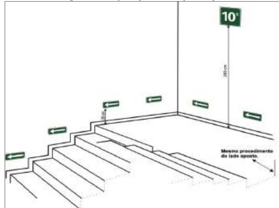
Figura 218. Sinalização complementar. Exemplo de rodapé
