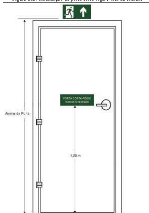
Figura 219. Sinalização de porta corta-fogo (vista da escada)
