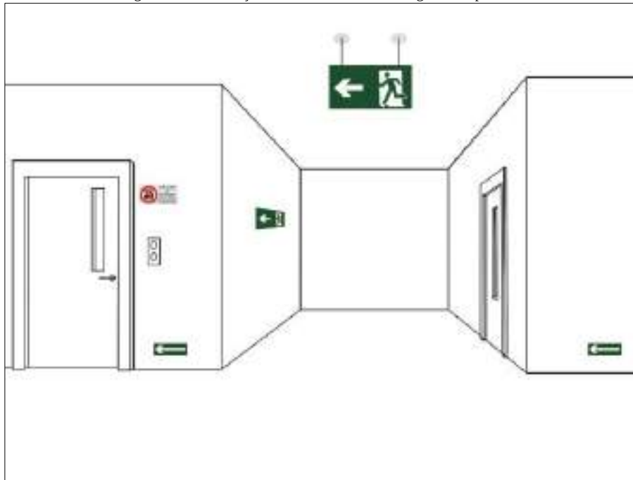
Figura 217. Sinalização de saída no sentido da fuga, em dupla face
