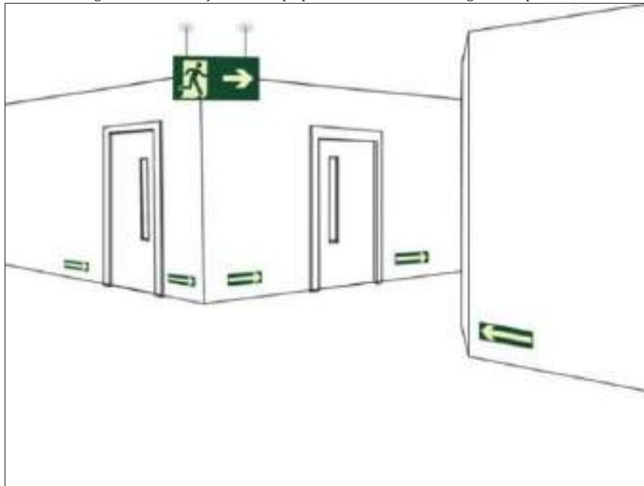
Figura 215. Sinalização de saída perpendicular ao sentido da fuga, em dupla face
