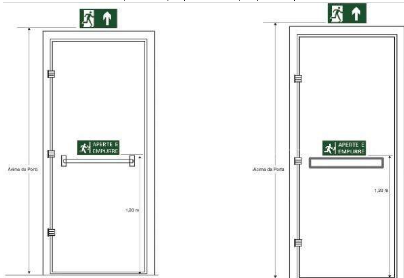
Figura 223. Sinalização de portas com barras antipânico (modelos 1 e 2)
