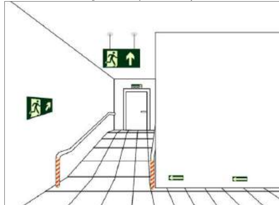
Figura 216. Sinalização de saída em rampa
