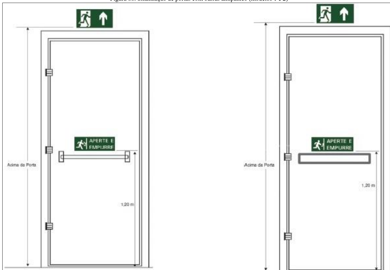
Figura 88. Sinalização de portas com barras antipânico (modelos 1 e 2)
