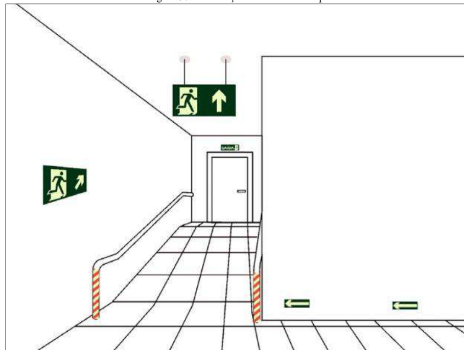
Figura 57. Sinalização de saída em rampa
