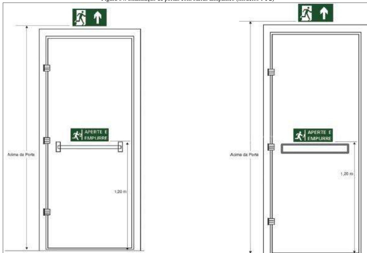
Figura 64. Sinalização de portas com barras antipânico (modelos 1 e 2)
