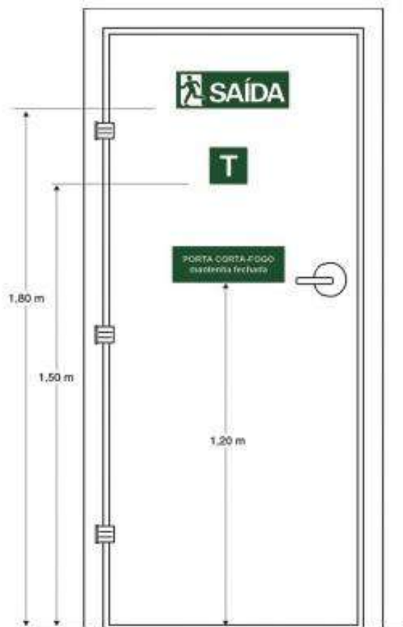
Figura 62. Sinalização de porta corta-fogo
