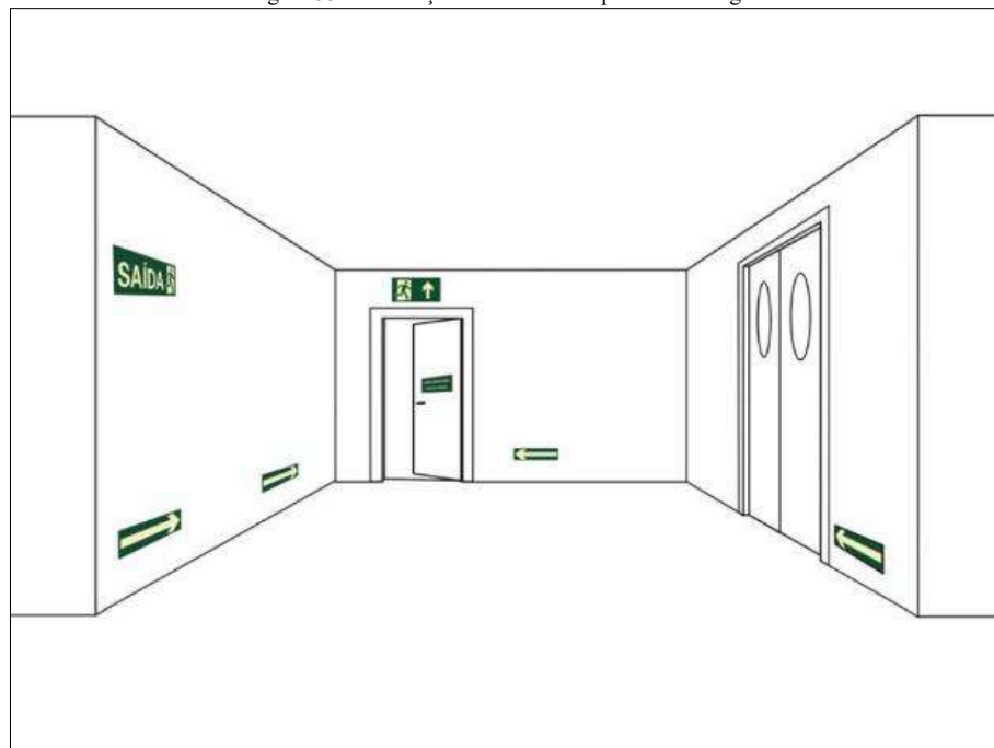
Figura 55. Sinalização de saída sobre porta corta-fogo
