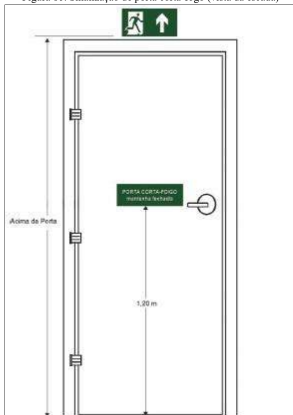
Figura 60. Sinalização de porta corta-fogo (vista da escada)
