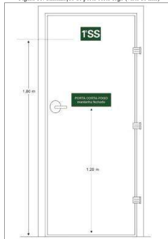
Figura 61. Sinalização de porta corta-fogo (vista do hall)
