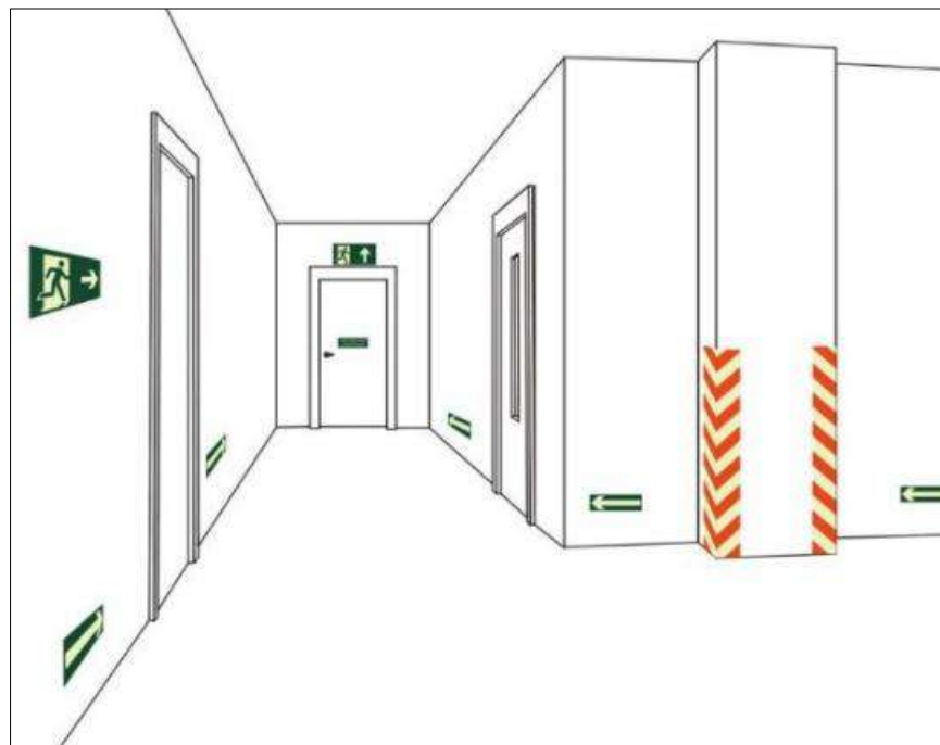
Figura 53. Sinalização de saída sobre porta corta-fogo - Sinalização complementar de saída e obstáculos
