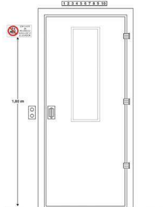
Figura 63. Sinalização de elevadores (vista da escada)
