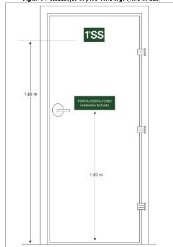
Figura 84. Sinalização de porta corta-fogo (vista do hall)
