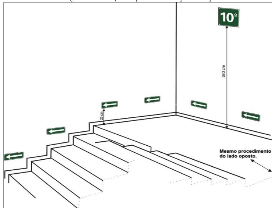
Figura 82. Sinalização complementar. Exemplo de rodapé
