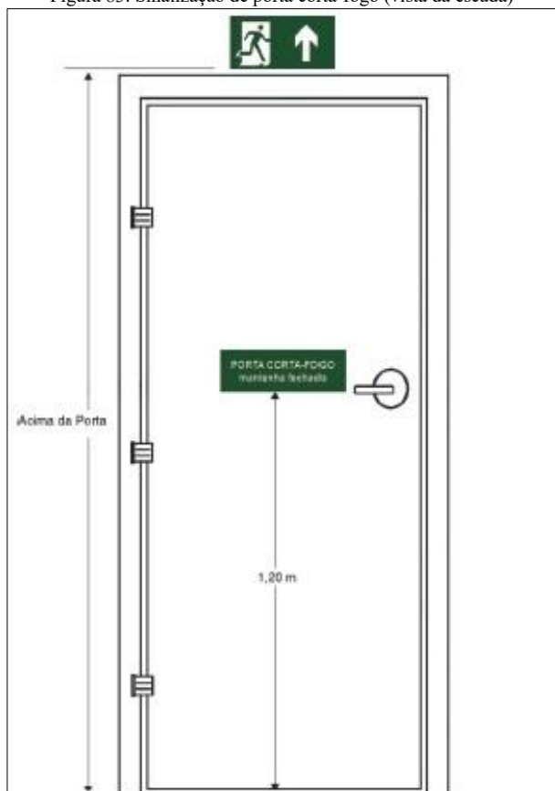
Figura 83. Sinalização de porta corta-fogo (vista da escada)
