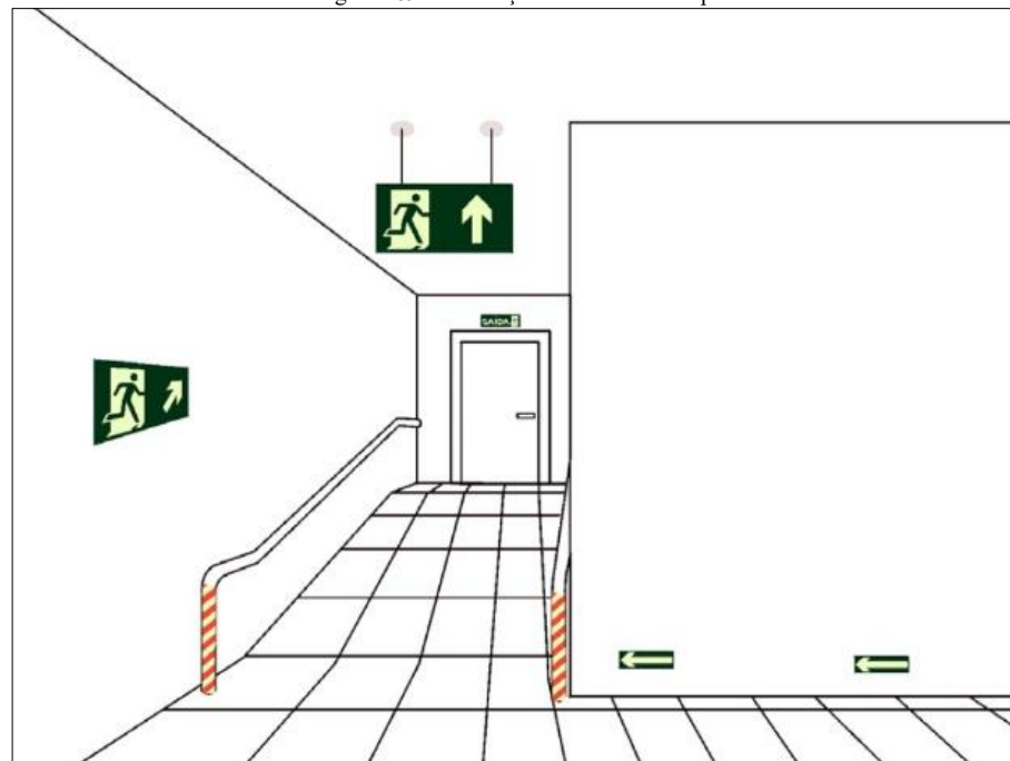
Figura 169. Sinalização de saída em rampa
