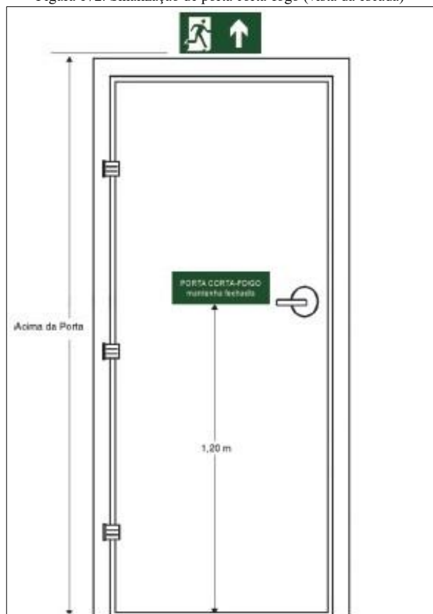
Figura 172. Sinalização de porta corta-fogo (vista da escada)
