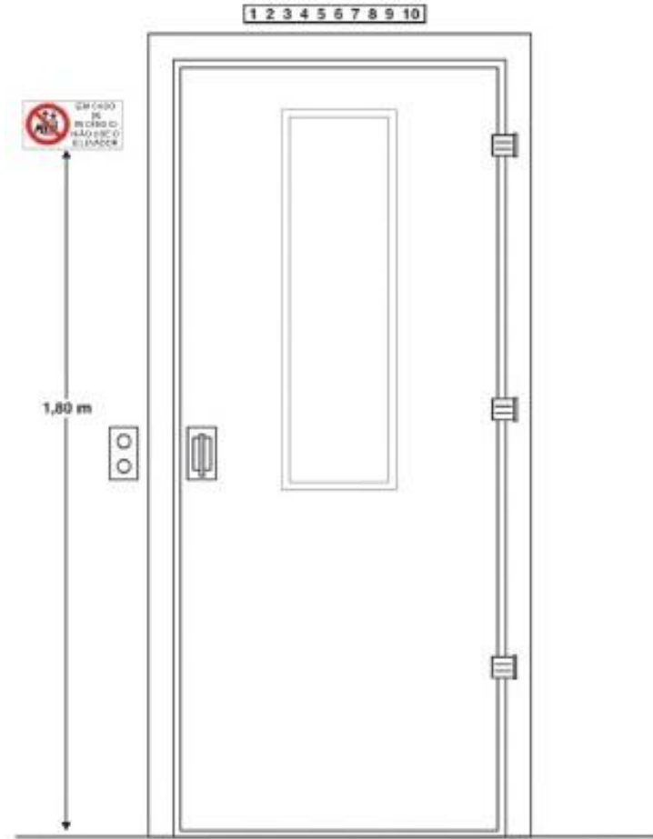
Figura 175. Sinalização de elevadores (vista da escada)
