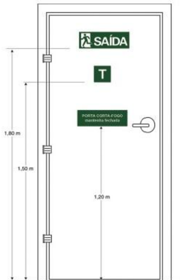
Figura 174. Sinalização de porta corta-fogo
