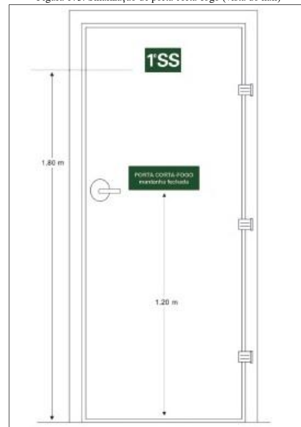
Figura 173. Sinalização de porta corta-fogo (vista do hall)
