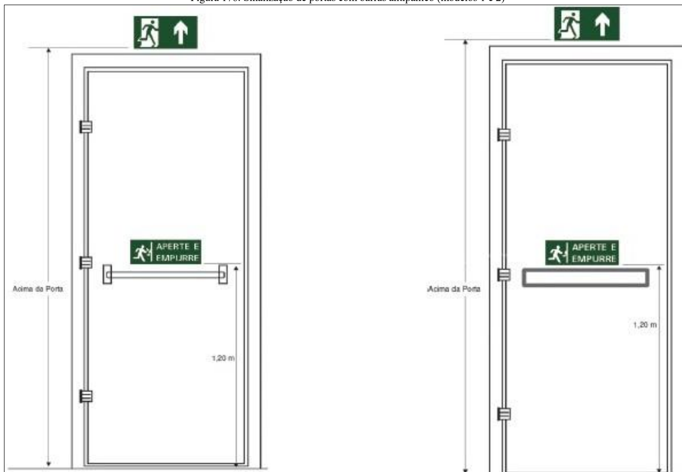
Figura 176. Sinalização de portas com barras antipânico (modelos 1 e 2)
