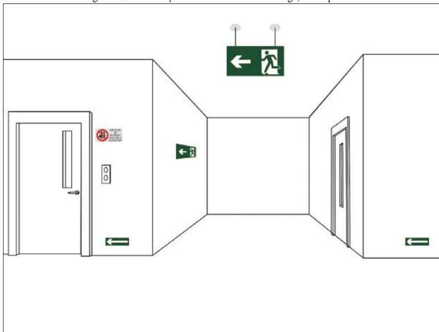
Figura 170. Sinalização de saída no sentido da fuga, em dupla face
