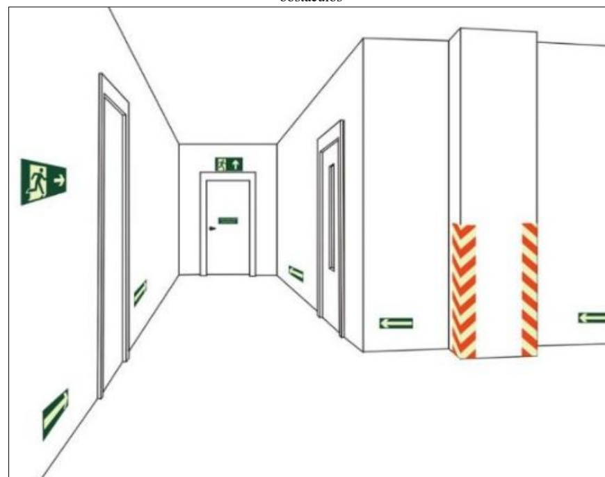
Figura 165. Sinalização de saída sobre porta corta-fogo - Sinalização complementar de saída e obstáculos
