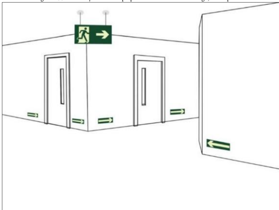
Figura 168. Sinalização de saída perpendicular ao sentido da fuga, em dupla face
