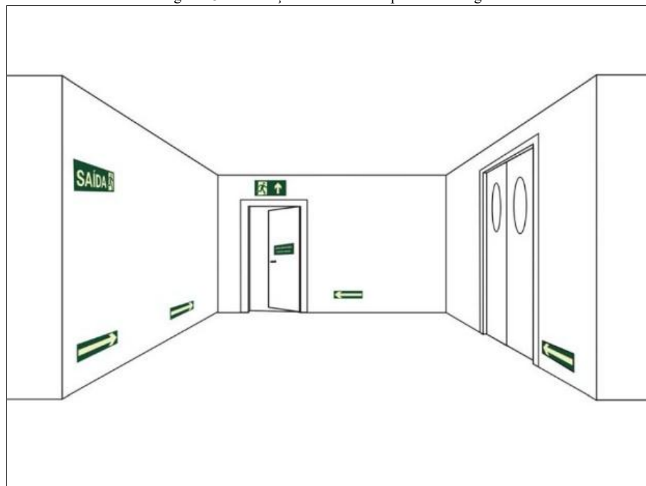
Figura 43. Sinalização de saída sobre porta corta-fogo
