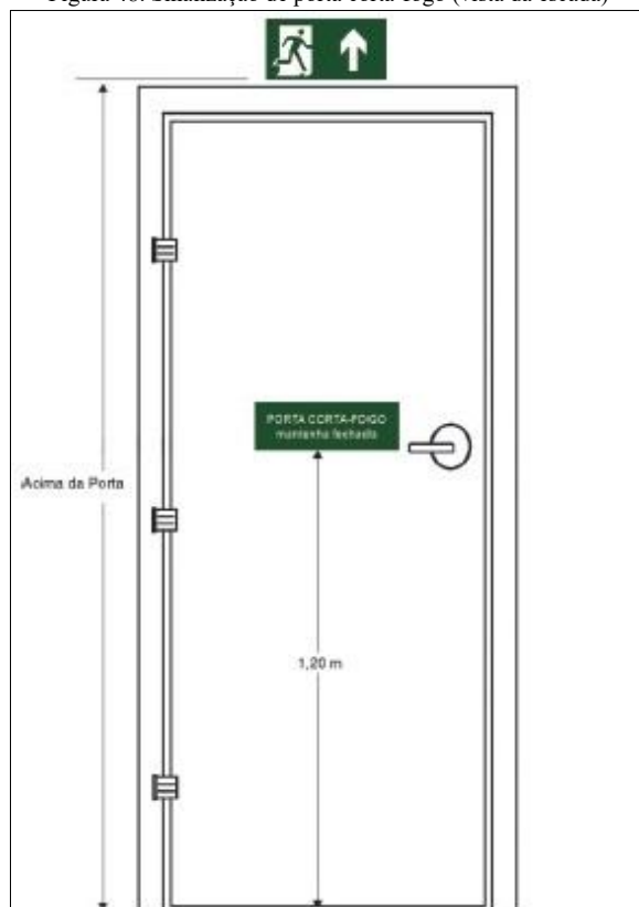
Figura 48. Sinalização de porta corta-fogo (vista da escada)
