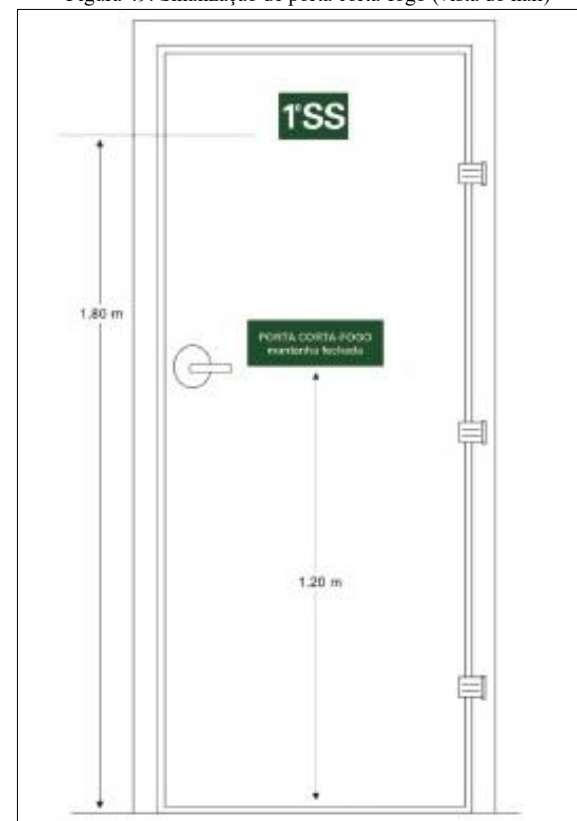
Figura 49. Sinalização de porta corta-fogo (vista do hall)
