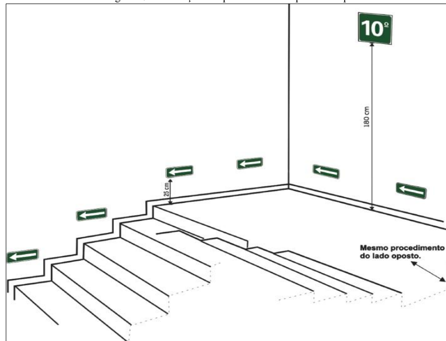
Figura 47. Sinalização complementar. Exemplo de rodapé
