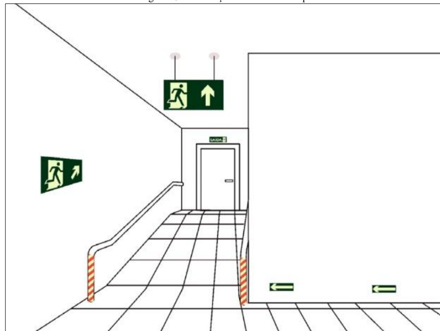
Figura 45. Sinalização de saída em rampa
