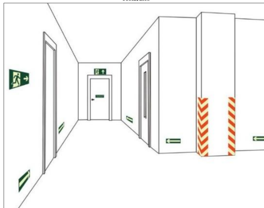
Figura 41. Sinalização de saída sobre porta corta-fogo - Sinalização complementar de saída e obstáculos
