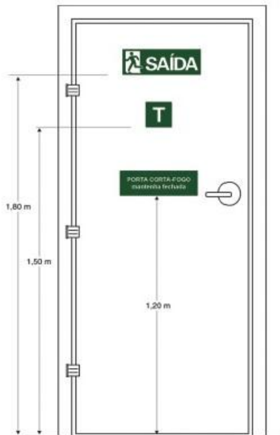
Figura 50. Sinalização de porta corta-fogo
