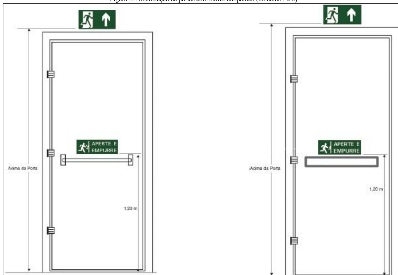
Figura 52. Sinalização de portas com barras antipânico (modelos 1 e 2)
