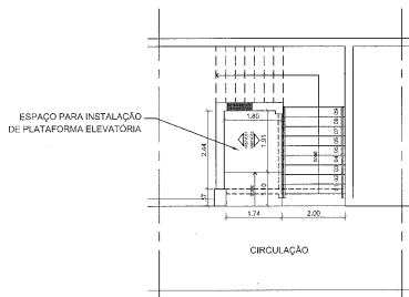
PLANTA DE REFORMA PAVIMENTO TÉRREO
