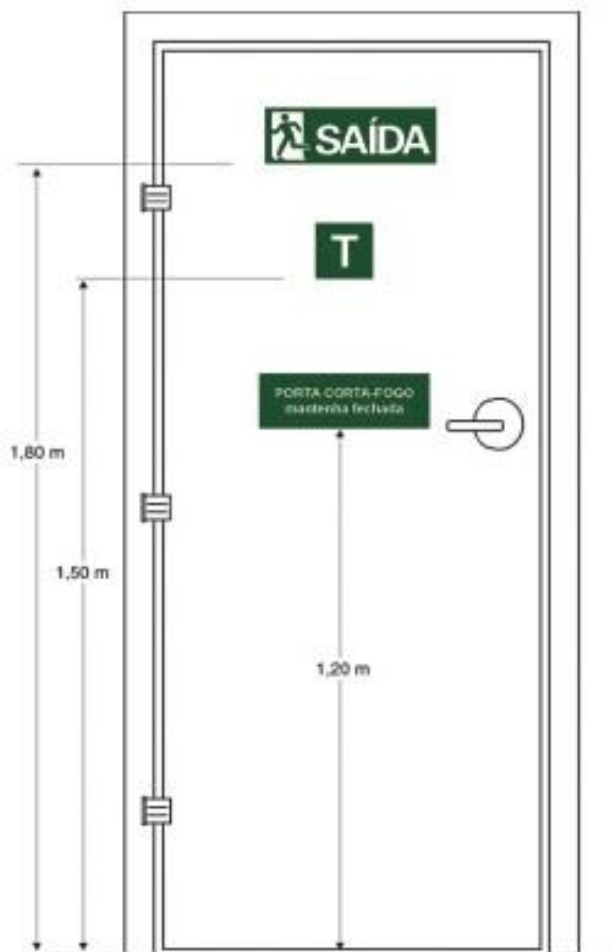
Figura 26. Sinalização de porta corta-fogo
