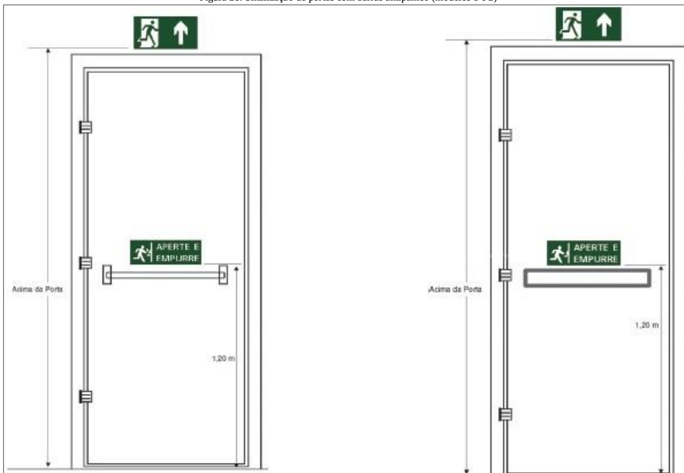
Figura 28. Sinalização de portas com barras antipânico (modelos 1 e 2)
