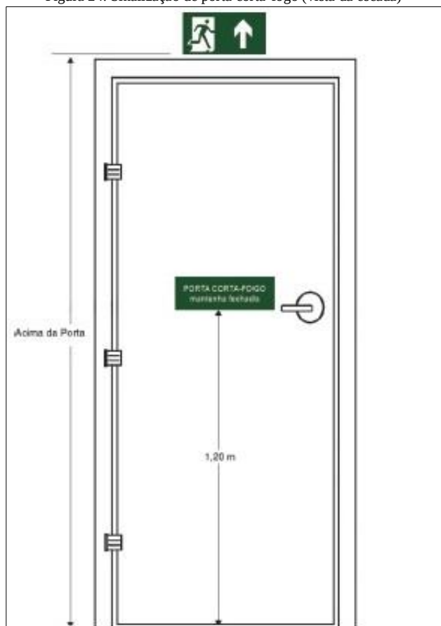
Figura 24. Sinalização de porta corta-fogo (vista da escada)
