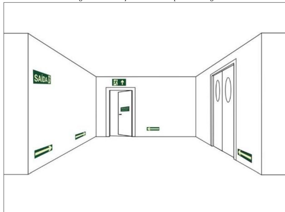
Figura 19. Sinalização de saída sobre porta corta-fogo
