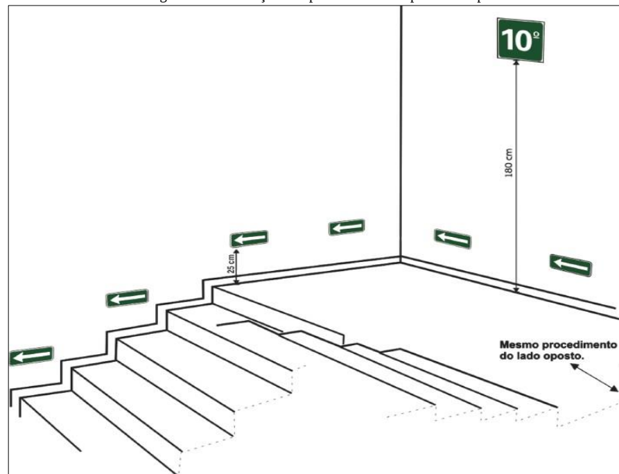
Figura 23. Sinalização complementar. Exemplo de rodapé
