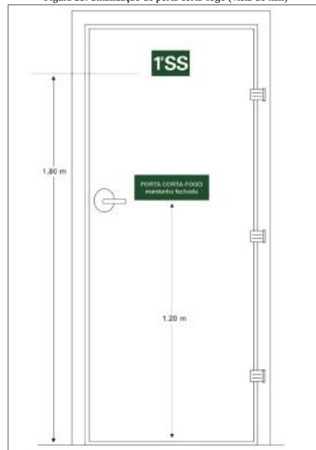
Figura 25. Sinalização de porta corta-fogo (vista do hall)
