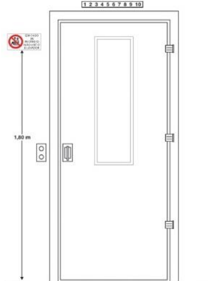
Figura 26. Sinalização de elevadores (vista da escada)
