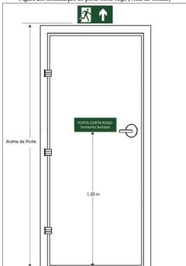
Figura 23. Sinalização de porta corta-fogo (vista da escada)
