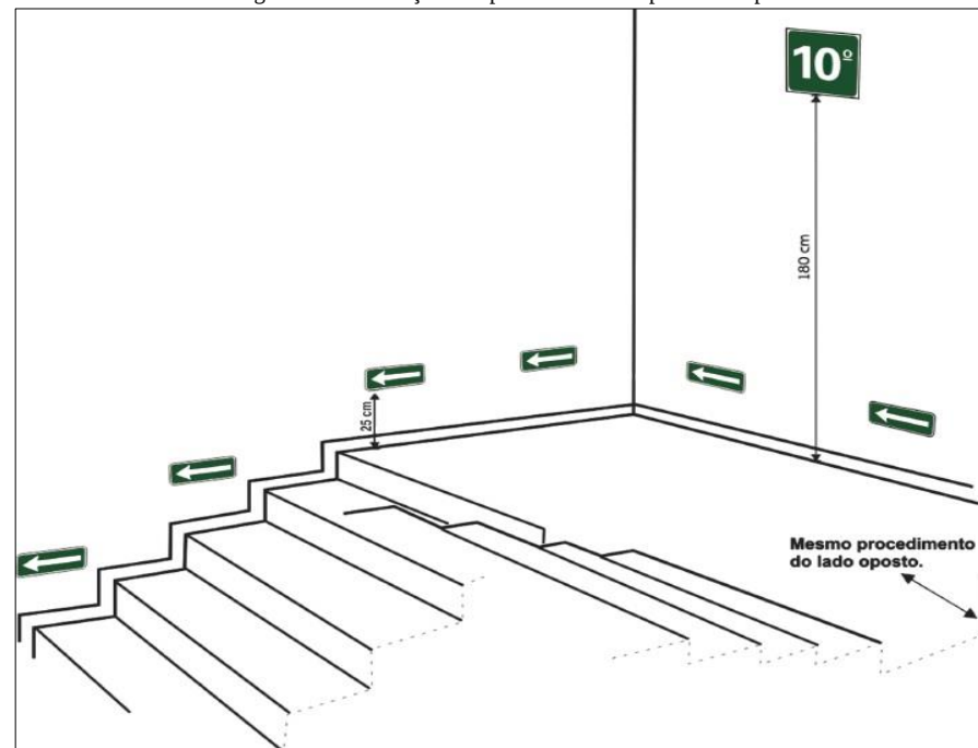
Figura 22. Sinalização complementar. Exemplo de rodapé
