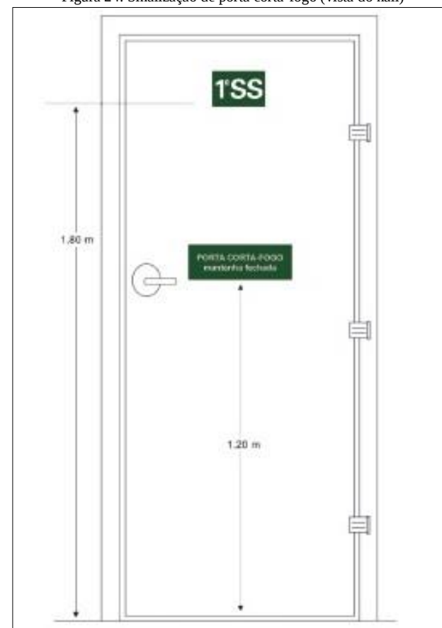
Figura 24. Sinalização de porta corta-fogo (vista do hall)
