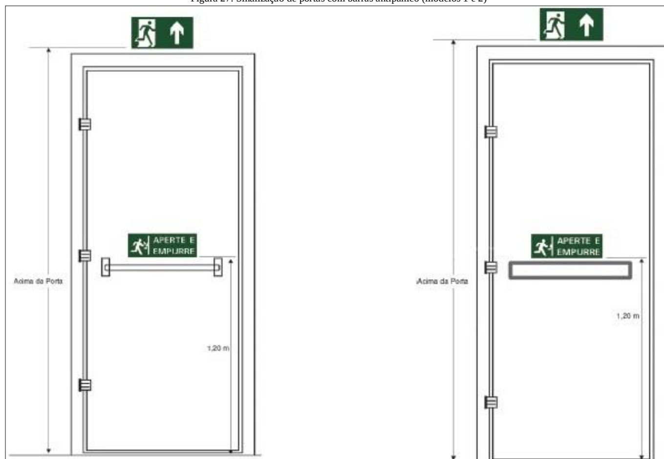
Figura 27. Sinalização de portas com barras antipânico (modelos 1 e 2)
