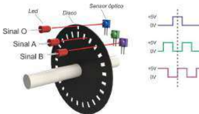
Figura 30: Exemplo de funcionamento de um encoder.
