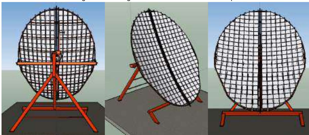
Figura 2: Modelagem do Concentrador em SketchUp.
