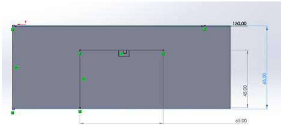
Figura 25 - Esboço do projeto
