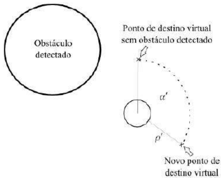
Figura 37: Funcionamento do controlador de evitar obstáculos
