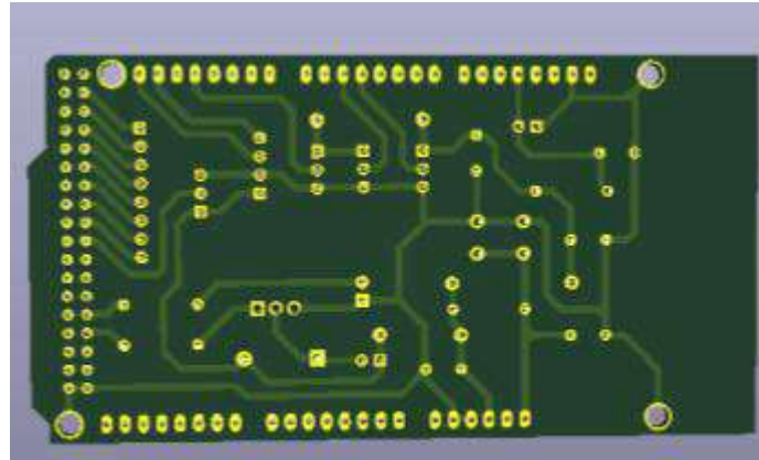
Figura 12 – Esquema da placa
