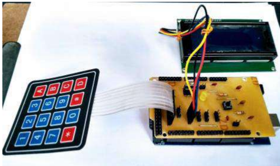
Figura 16: Estrutura construída.
