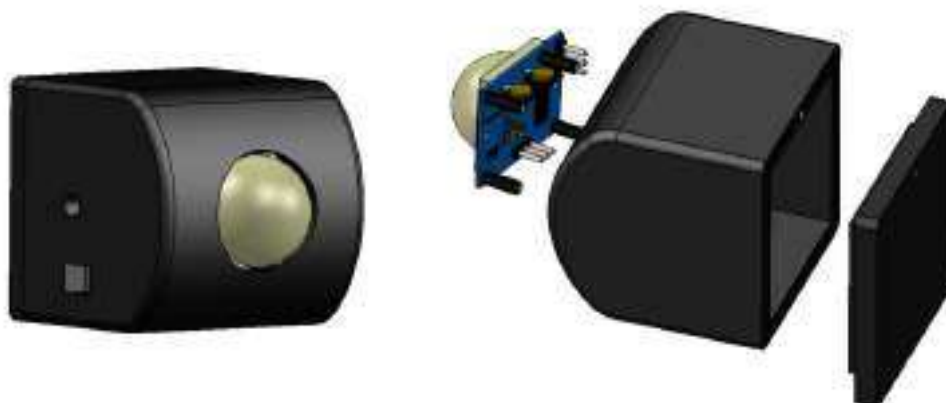
Figura 23 - Adaptação do sensor de presença
