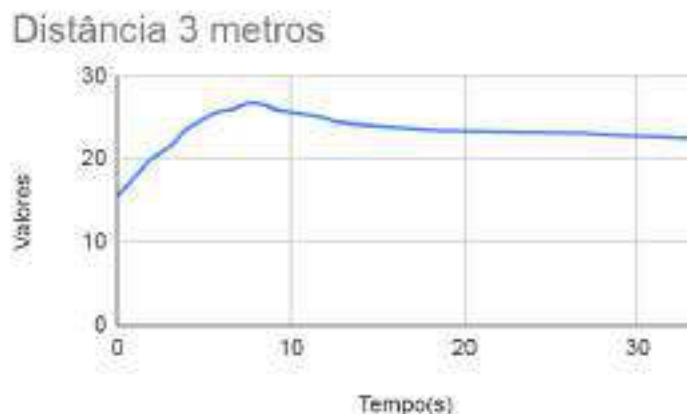
Figura 10 - Variação de radiação UVC com com 2 lâmpadas ligadas.
