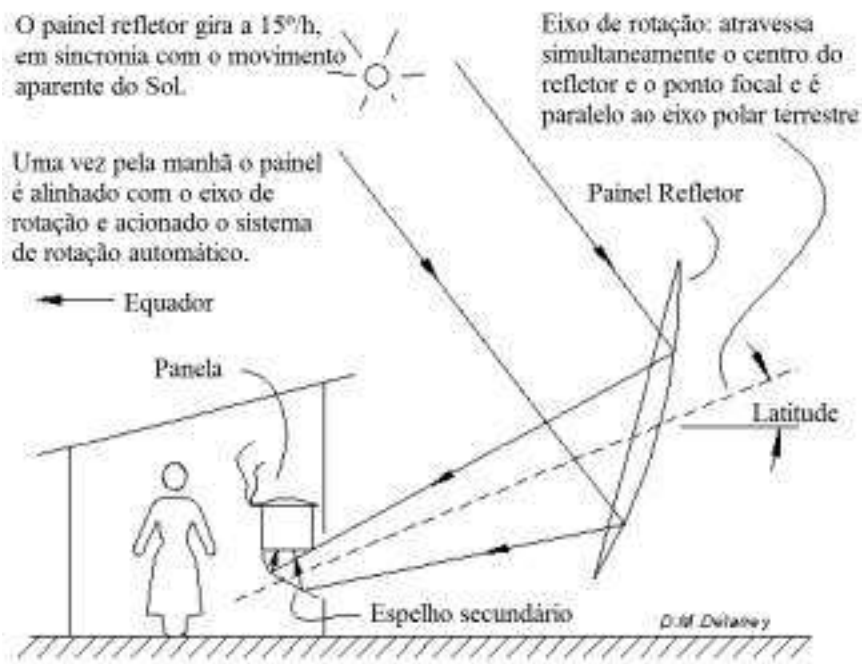
Figura 1: Esquema Básico do Concentrador de Scheffler
