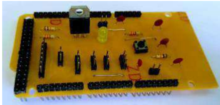
Figura 15: Placa finalizada
