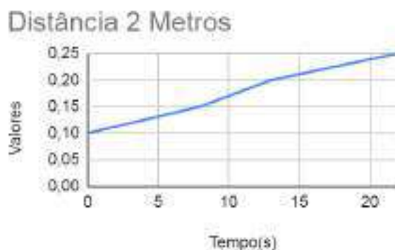
Figura 9 - Variação de radiação UVC com com 2 lâmpadas ligadas.
